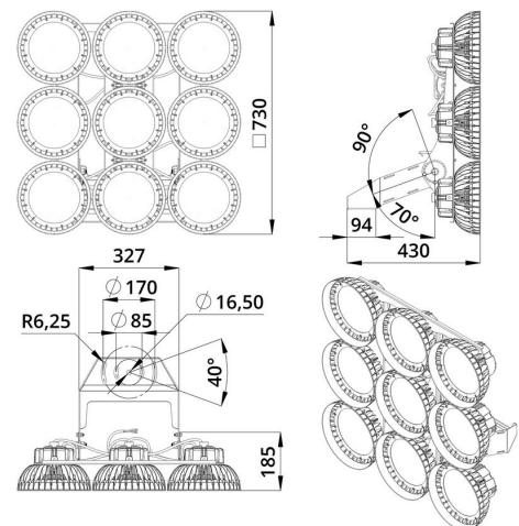
Габаритный чертеж
