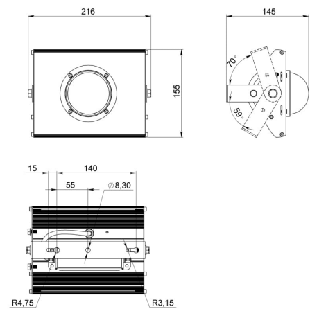
Габаритный чертёж
